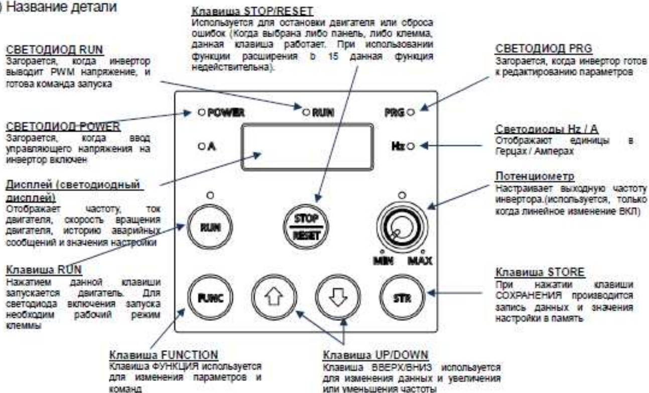
Рис.1 Панель светодиодного типа
